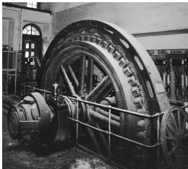
Gaswerk Schlieren, MFO Generator der Sulzer Dampfmaschine 1904, Hans-Peter Bärtschi 1998, e-pics.ethz.ch
